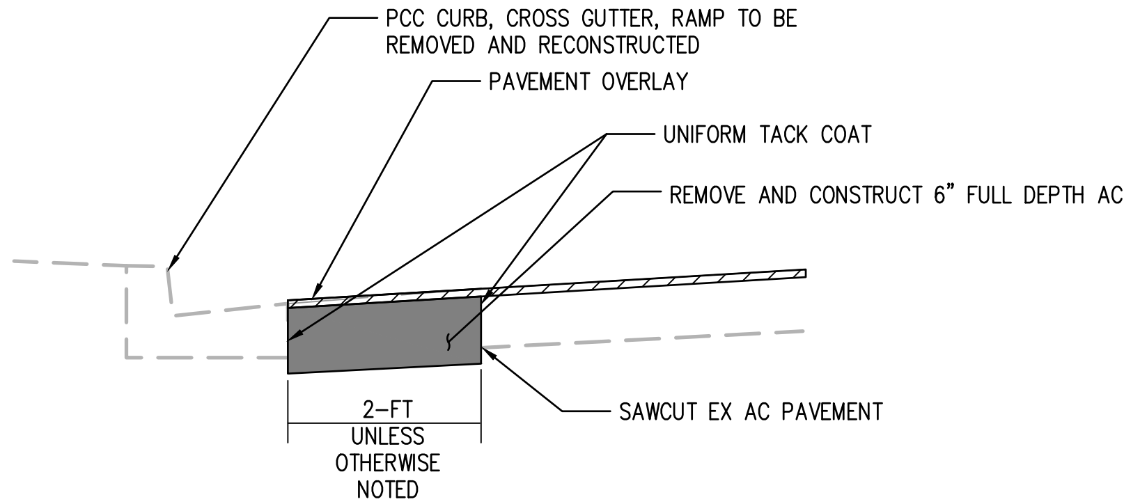
SLOT PAVEMENT DETAIL "1" N.T.S.
